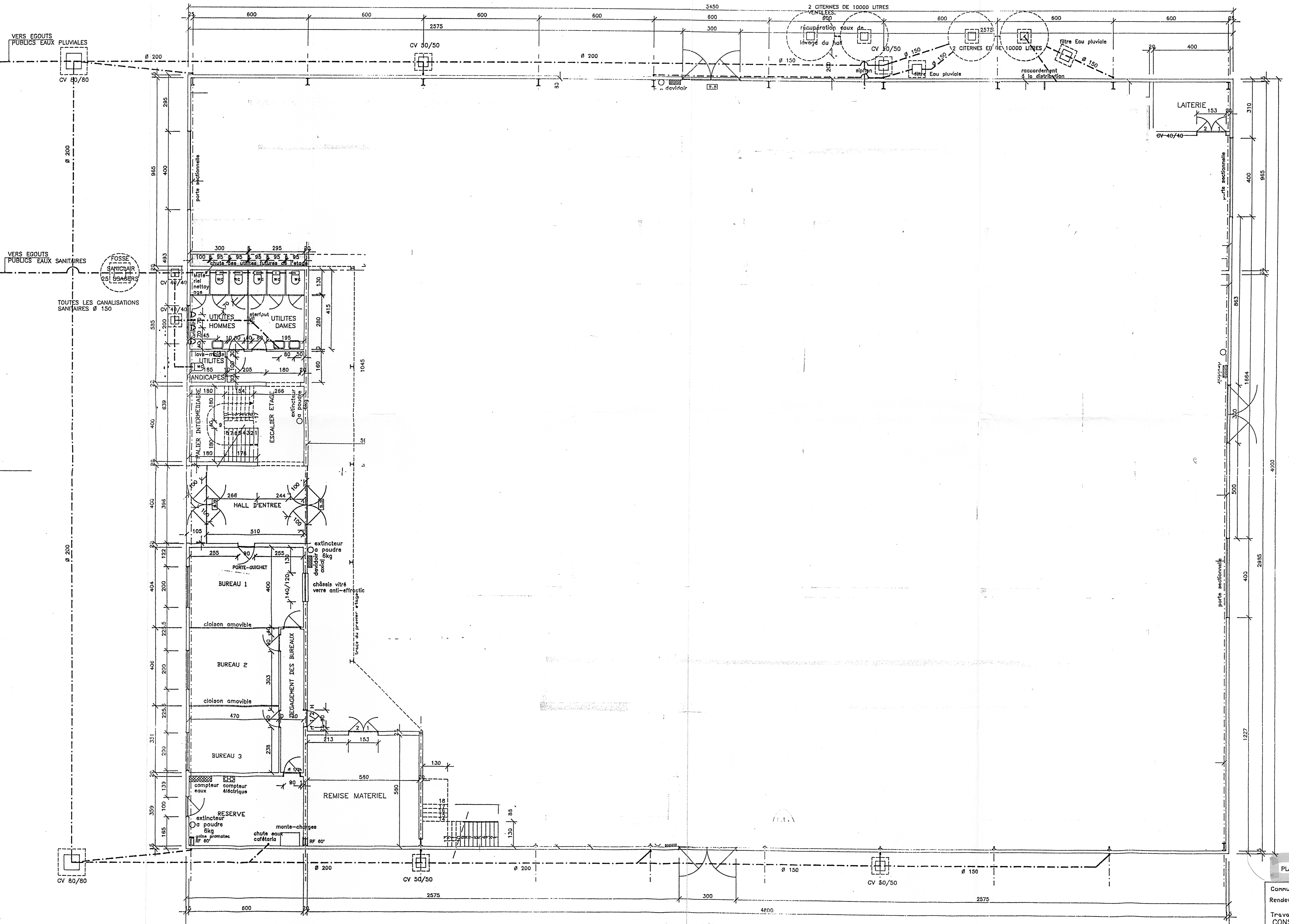
PLAN DU REZ-DE-CHAUSSEE ECHELLE 1/100
